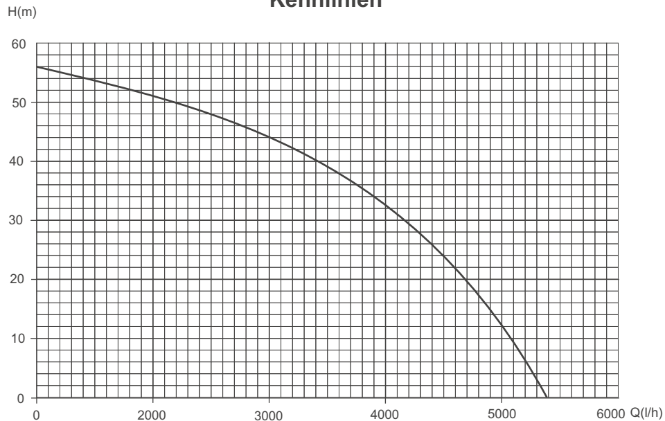
Kennlinien
